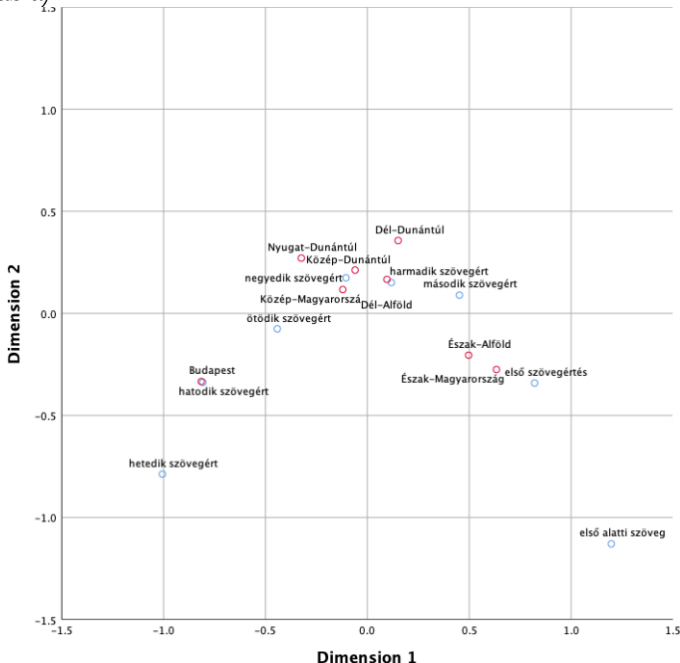
2. ábra: A magyarországi régiók és a kompetenciamérés során elérhető szövegértés szintek 2 dimenzióan ábrázolt szimmetrikus normalizációs ábrája a hatodik évfolyamos diákok esetében
